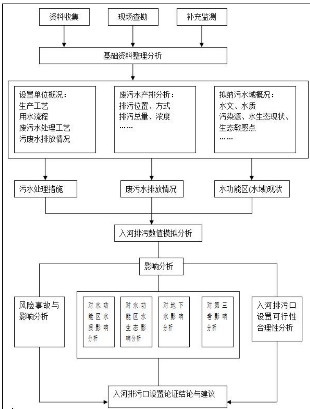
图 1.4-1 大村甸镇污水处理厂排污口分析工作程序
