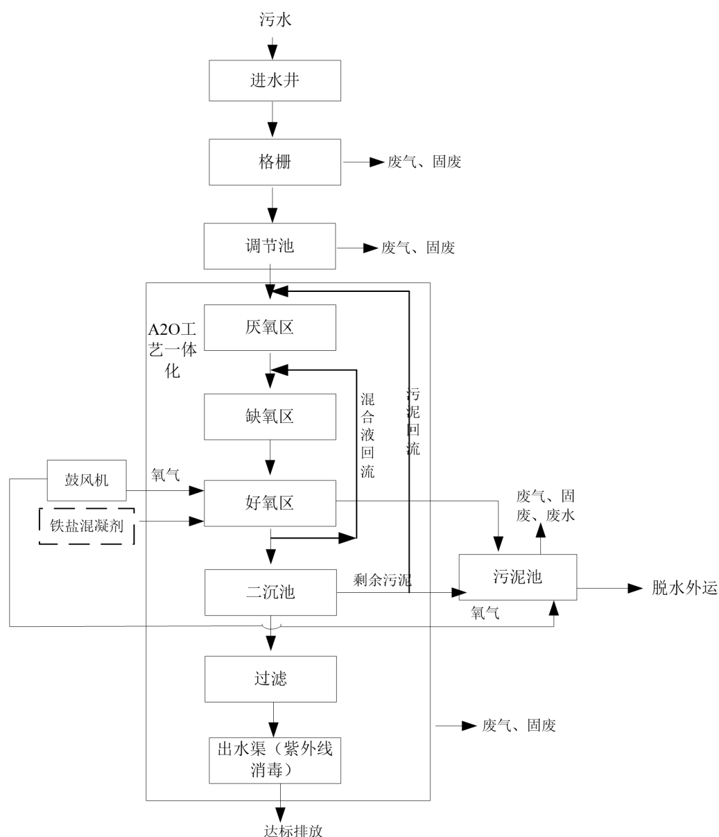
图 2.2-1 大村甸镇污水处理厂工艺流程及产污环节图
