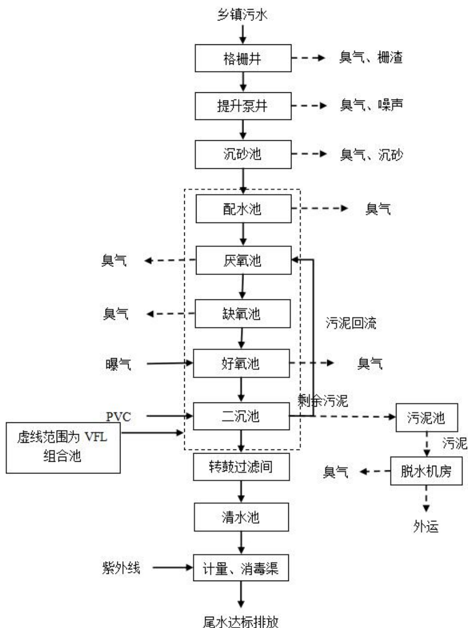
图 2.2-1 龚家坪镇污水处理厂工艺流程及产污环节图
