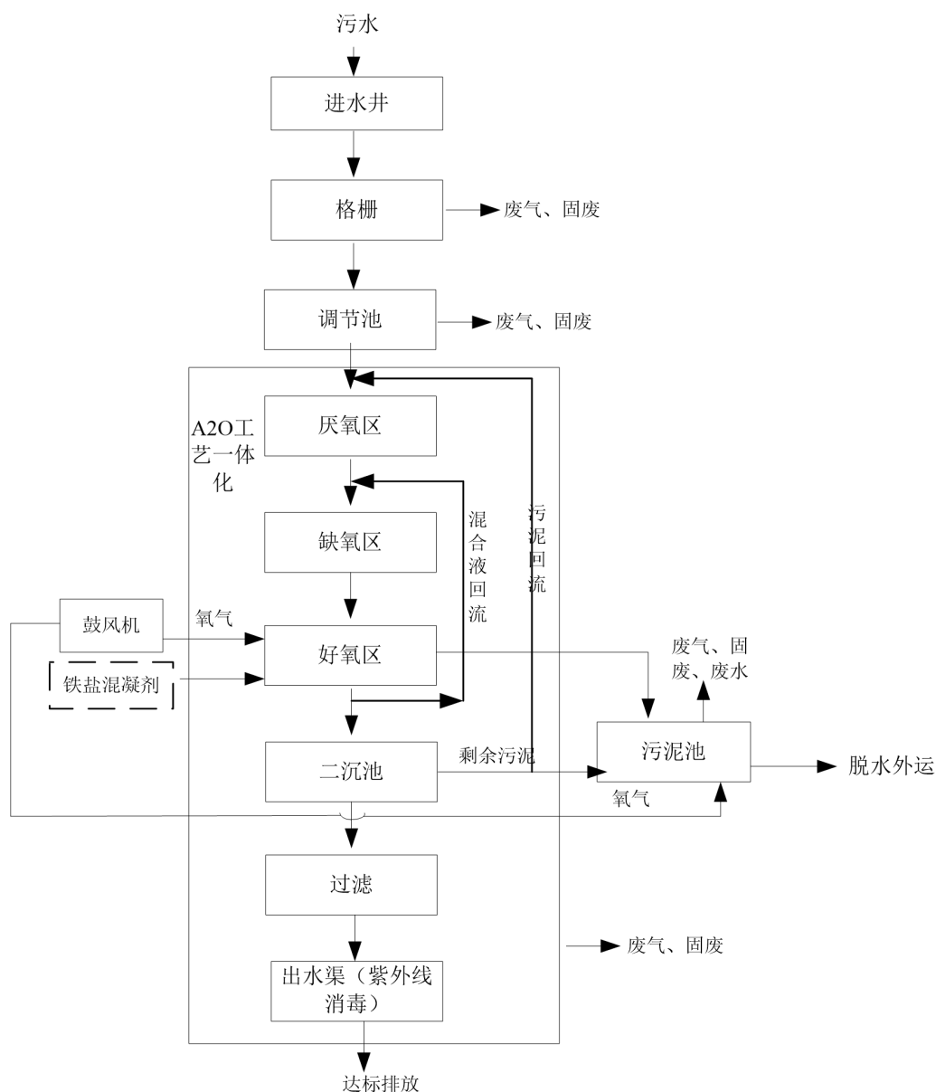
图 2.2-1 梅溪镇污水处理厂工艺流程及产污环节图
