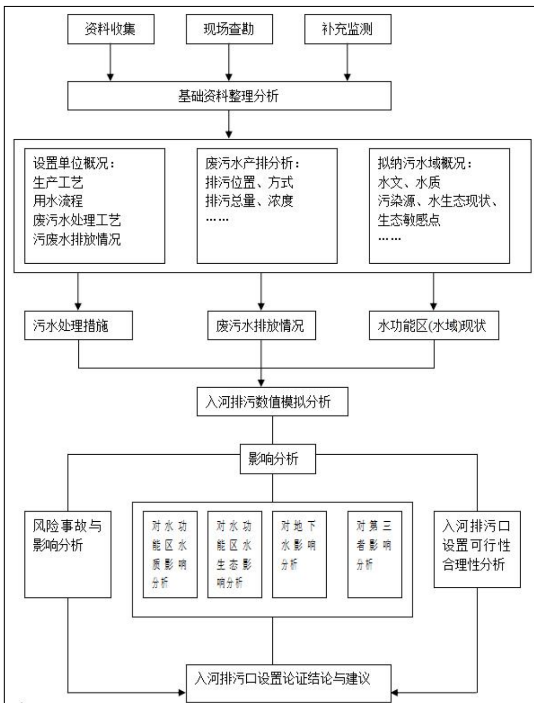
图 1.5-1 梅溪镇污水处理厂排污口分析工作程序
