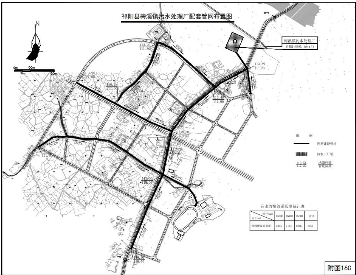
图 4.1-1 纳污范围图
