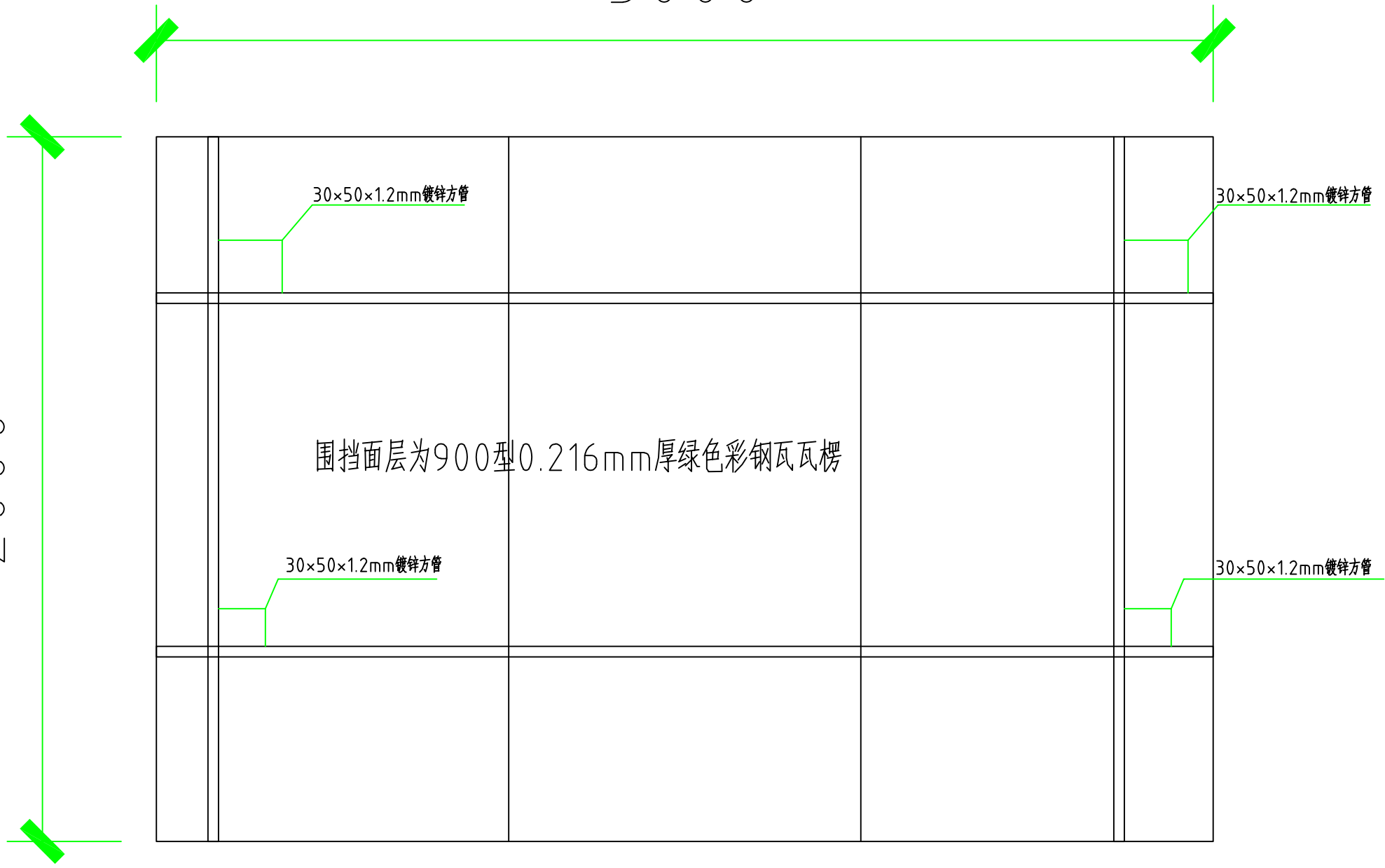
围挡平面图
