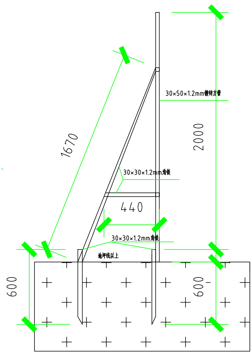
围挡基础图
