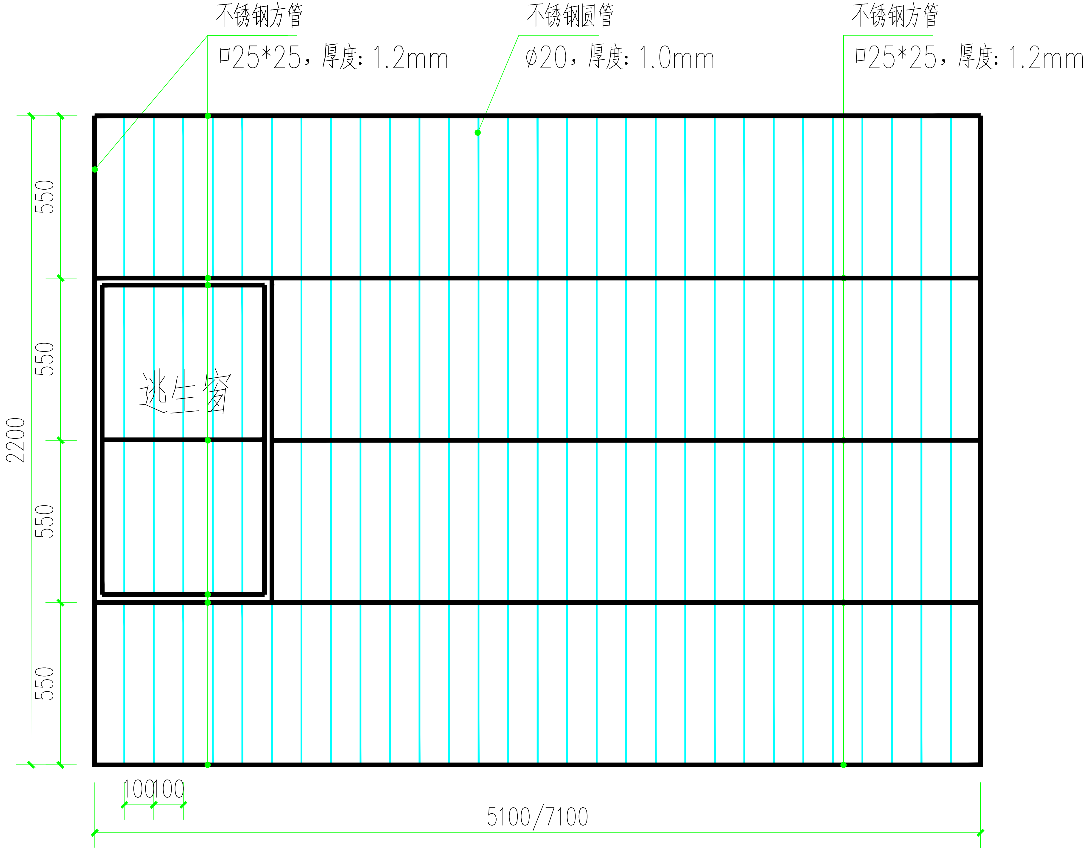
不锈钢防护网大样图 1:20
