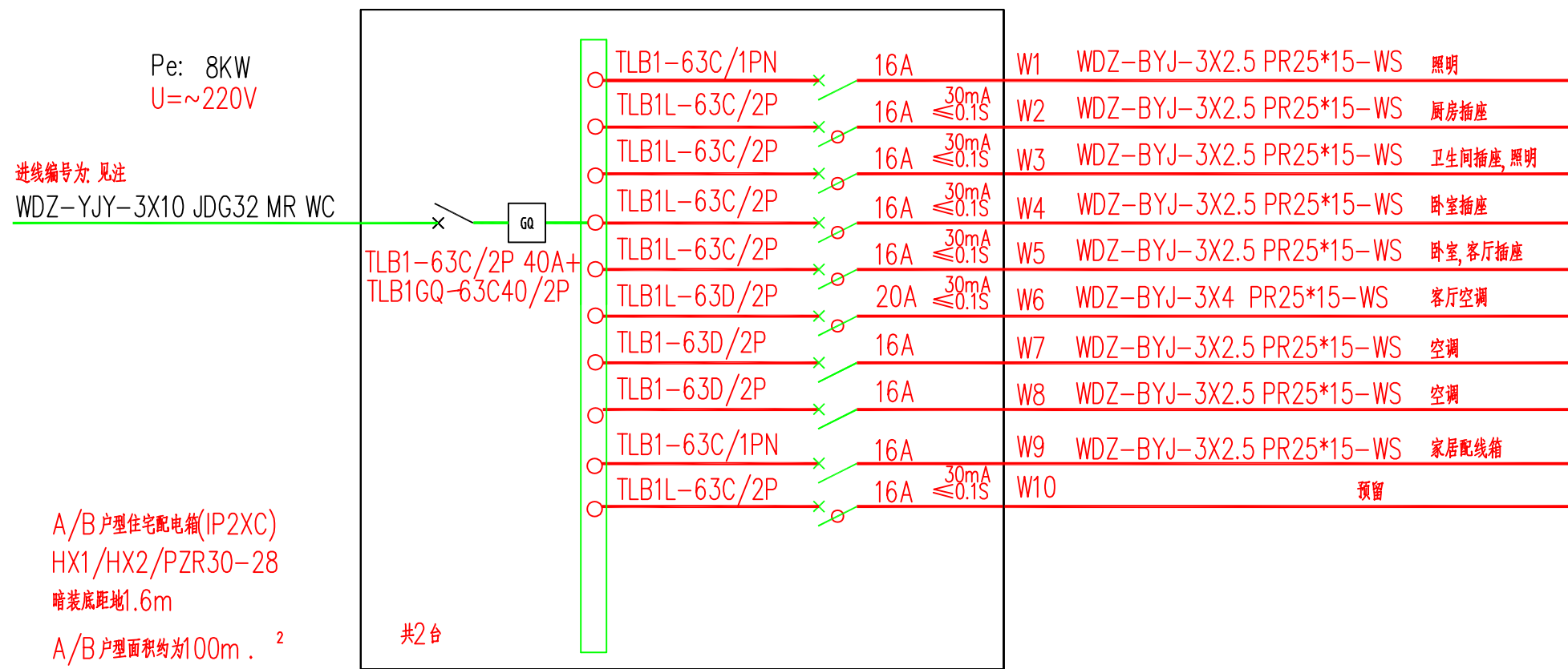
强电箱系统图
